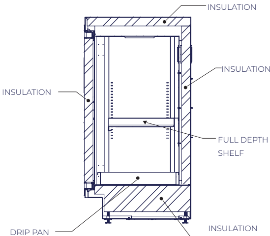
18-3/8" ACTUAL DEPTH
